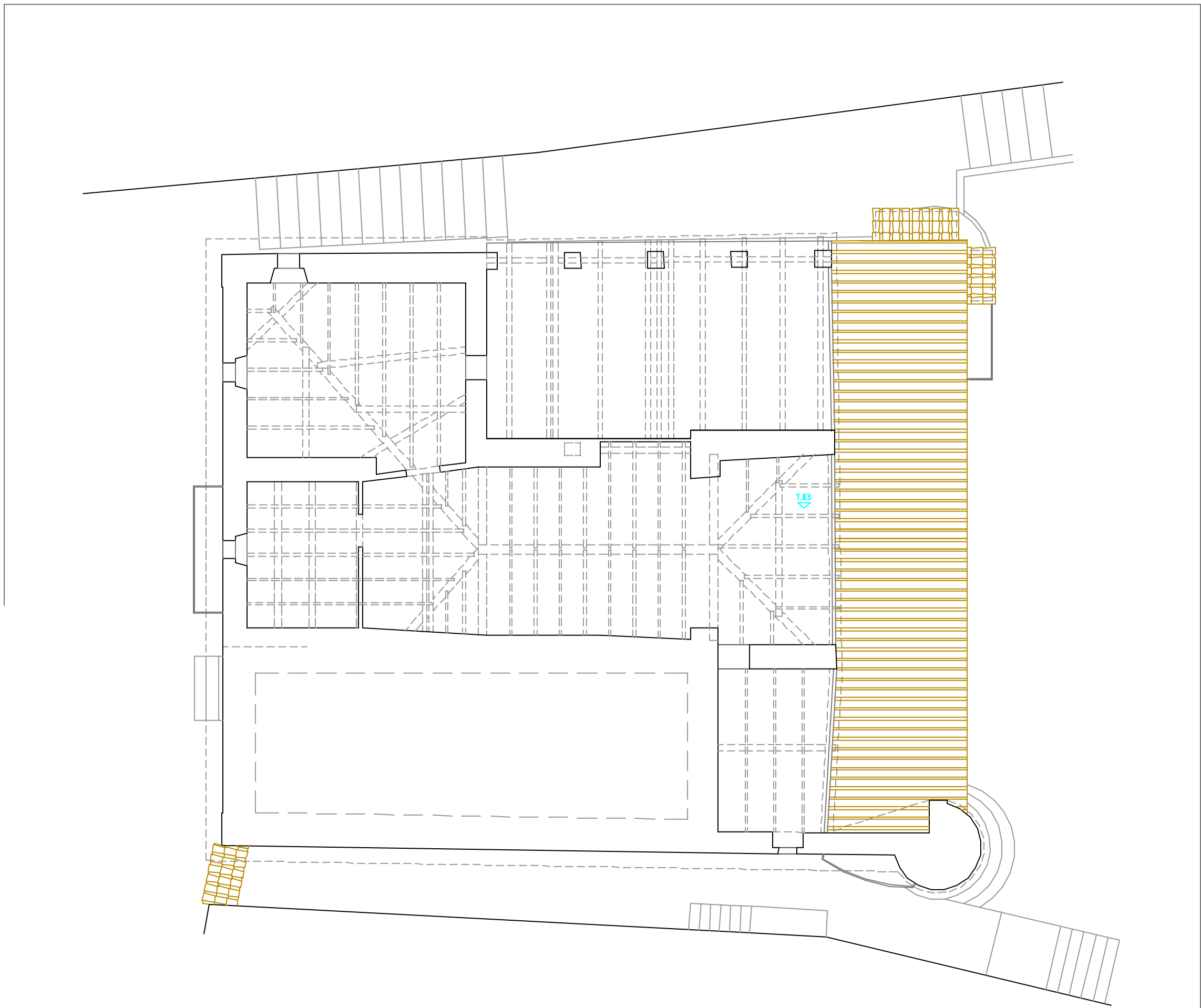
Pianta Piano Sottotetto
