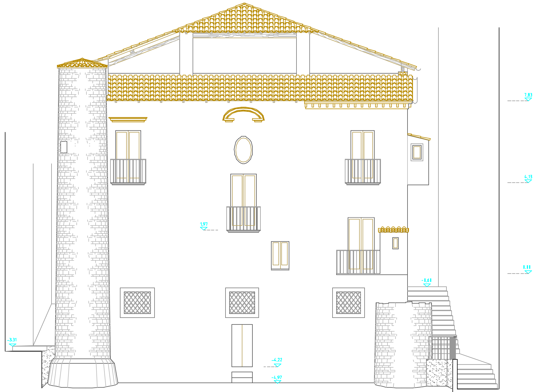
Prospetto Posteriore
