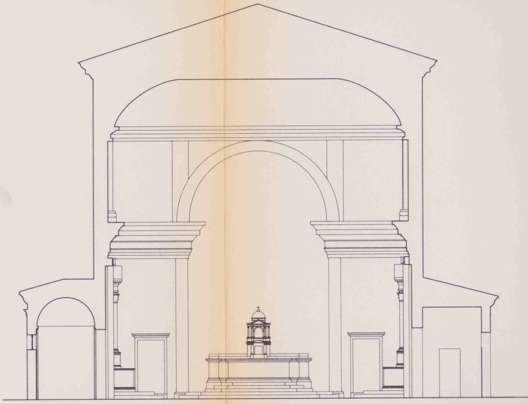
SEZIONE
