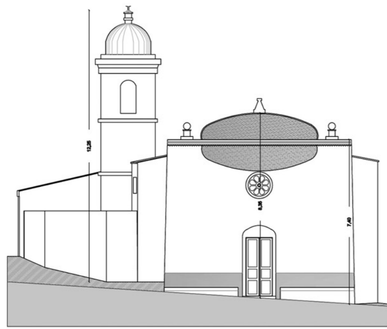
prospetto ovest
