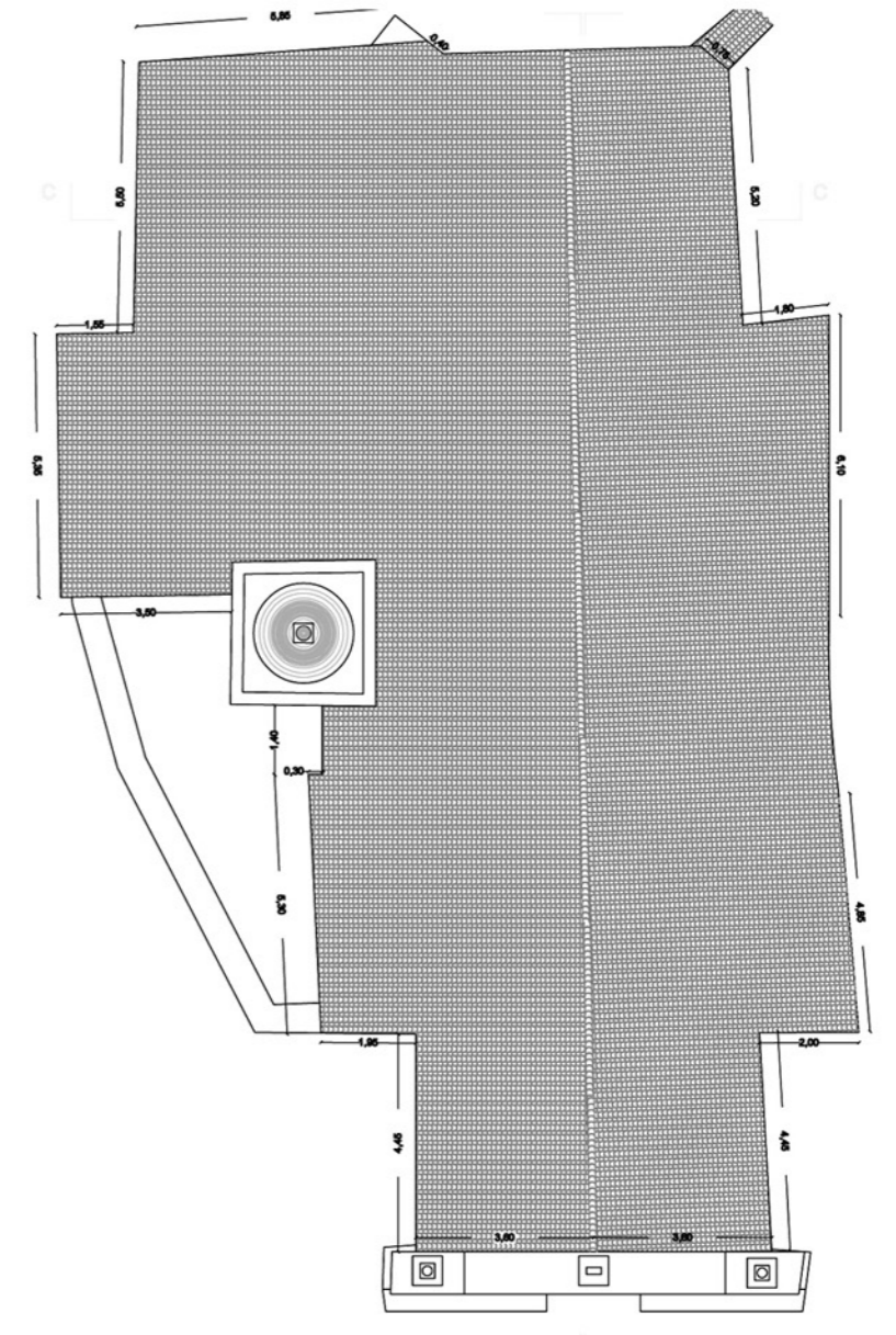
PIANTA CUPOLA
