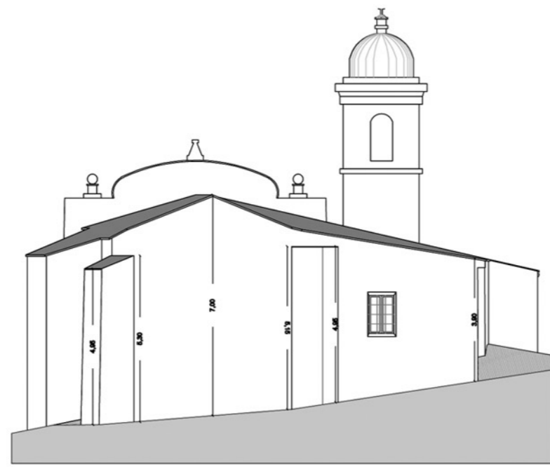
prospetto est
