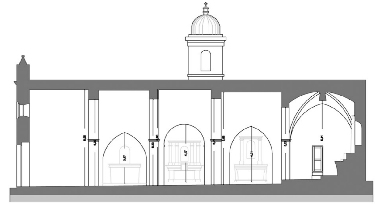
sezione longitudinale ovest-est
