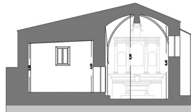
sezione trasversale
