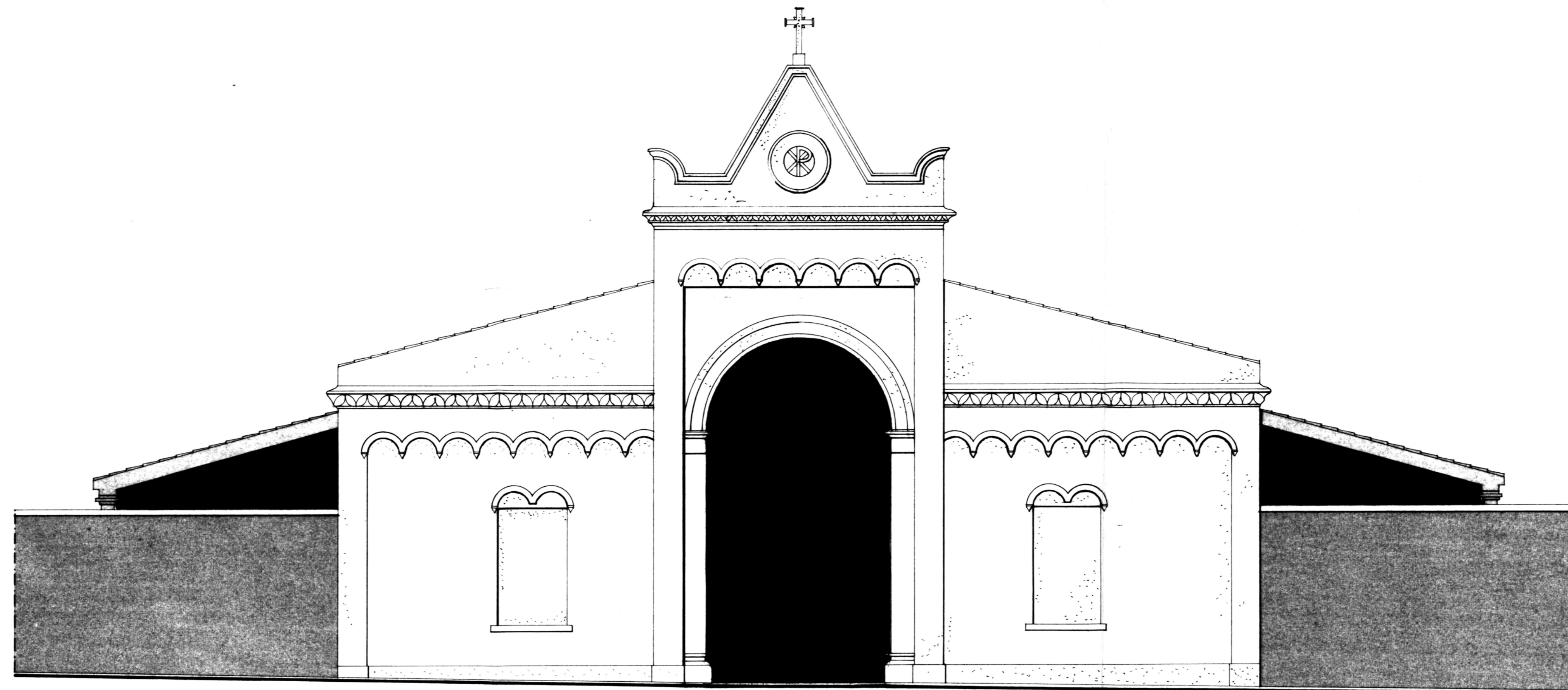
Prospetto esterno ingresso principale
