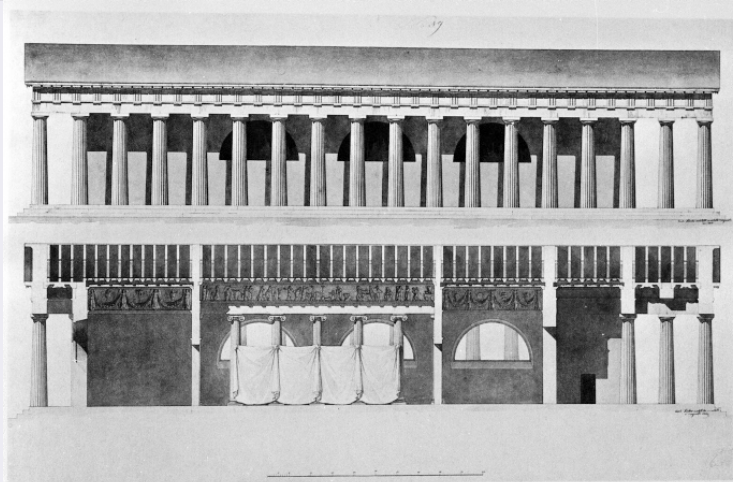
Walhalla, Aufriß Seitenfassade und Längsschnitt Entwurf II, 9.6
