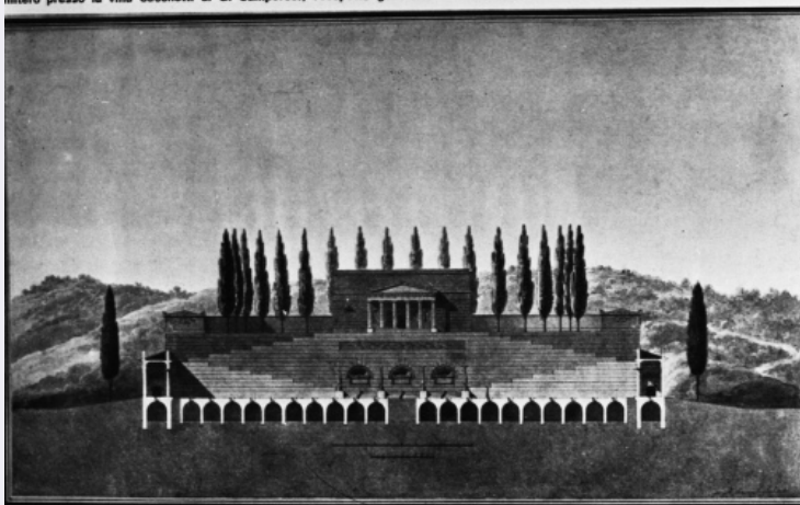
XXXV) In Archivio del conte C. de Tournon nel castello di Avrilly. Progetto per il cimitero presso la villa Sacchetti di G. Camporesi; Sezione longitudinale che fa vedere l'izato e la forma delle cripte.
