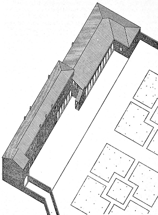
Fig. 19) Ipotesi di ricostruzione grafica, sulla base di fonti iconografiche e d'archivio, della parete Nord del complesso di Schifanoia, come doveva apparire dopo gli ultimi lavori di ampliamento del 1493.
