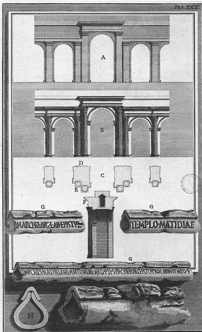
A et B Orthographia utriusque lateris arcuum ductus Aquae Virginis a specu principe ad Hadriani the- mas, offessorum prope aedem S. Ignatii. C Ichnographia eorumdem arcuum. D denotat vestigia lateris orthographici A. E denotat vestigia lateris orthographici B. F Sectio ipsorum arcuum. G Fragmenta tu- borum plumbearum. H Area seu lumen eorumdem cum forma tegumenti summae juncturae: quae hactenus reperta sunt.
