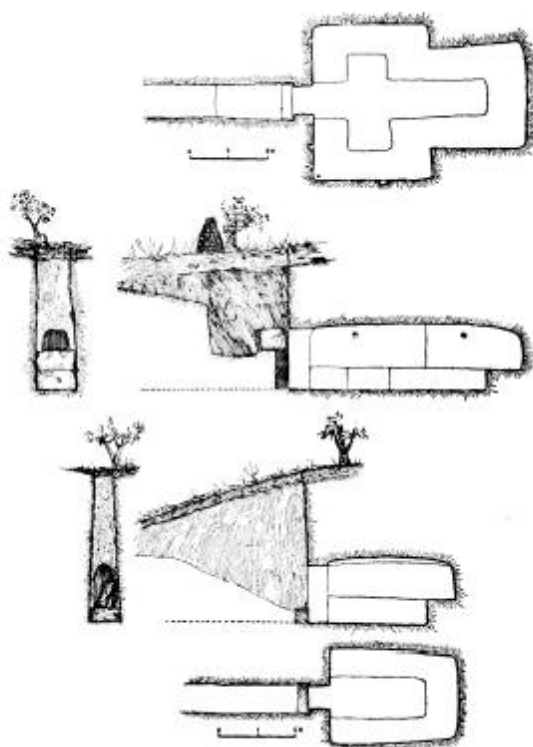
FIG. 5. — PLANS ET SECTIONS DES TOMBES IX ET V
