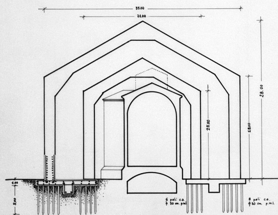
ARMATURA DEI PORTALI SOPRA MAGLIA SUPERFICIALE (CINE' INTERAMENTE IN ALLUMINIO) (CINQUE A LA MIRA 15 CM. DI STRATTO 8/24) SCALA 1:1000
