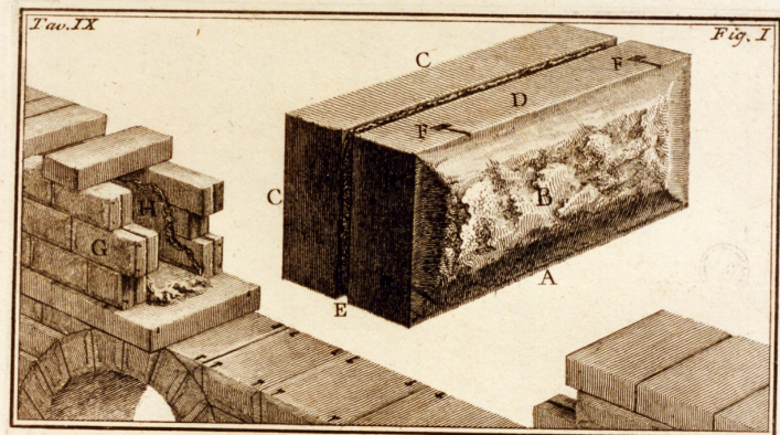
Tav. IX Fig. I A. Pezzo di tufo. B. Parte esterna. C. Lato interno. D. Lati, che connettevano con gli altri pezzi. E. Canale ripieno di lastrico. F. Burchi per i perni. Per maggior chiarezza poi del suddetto pezzo è mostrato come doveva stare in opera nel suo acquedotto G. H. Condotto G. H. Condotto Francesco Arcoletto del. inc.
