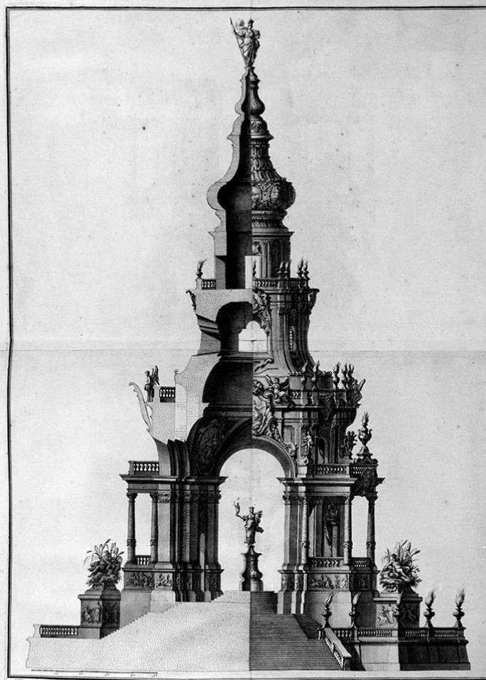
Disegno e Spaccato geometrico della Macchina del Fuoco d'artificio posta su la gran Piazza del Castello S. Pio. Piranesi del. Panzeri sculp.
